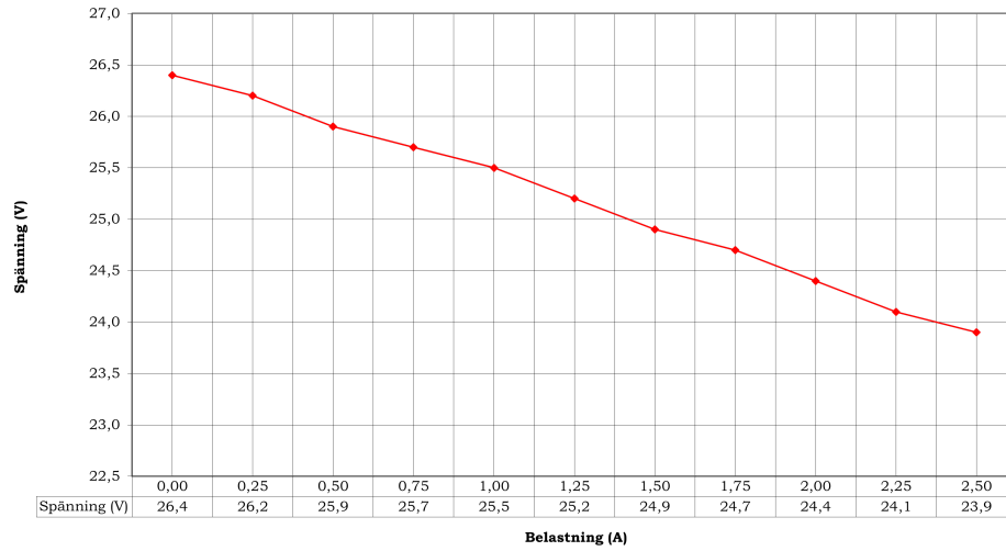
Belastningskaraktistik 6024-0177 PSS 60 230/24V
